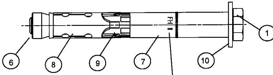
Schraubenversion Typ S FH II 12 - 32
