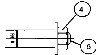
Gewindebolzenversion Typ B FH II 12 - 32
