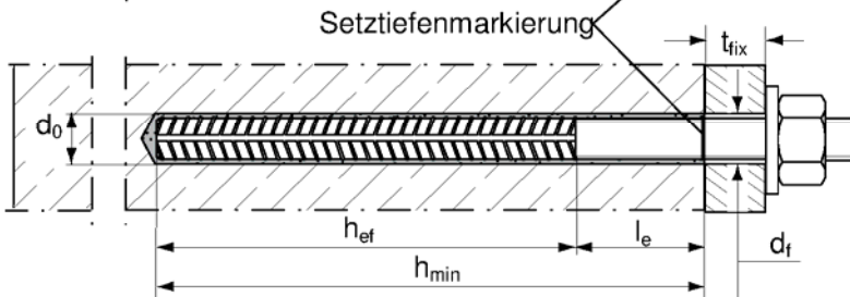
fischer Bewehrungs- Anker FRA
